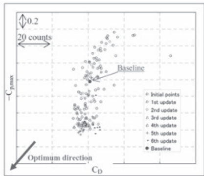
(a) CD - -C_{p,max}
