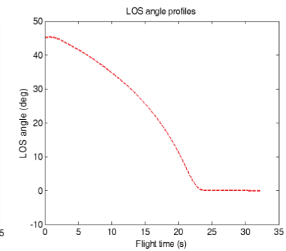
Fig. 11. LOS angle profile
